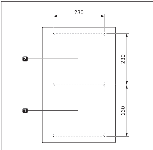
Afb. 4.7 Afmetingen kookzones
