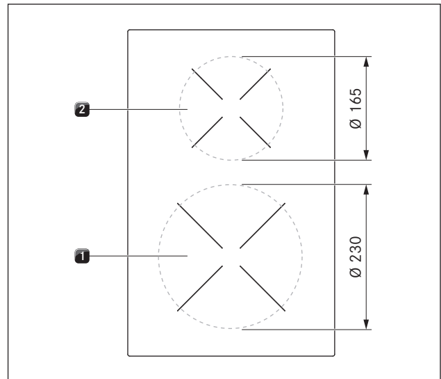
Afb. 4.9 Afmetingen kookzones
