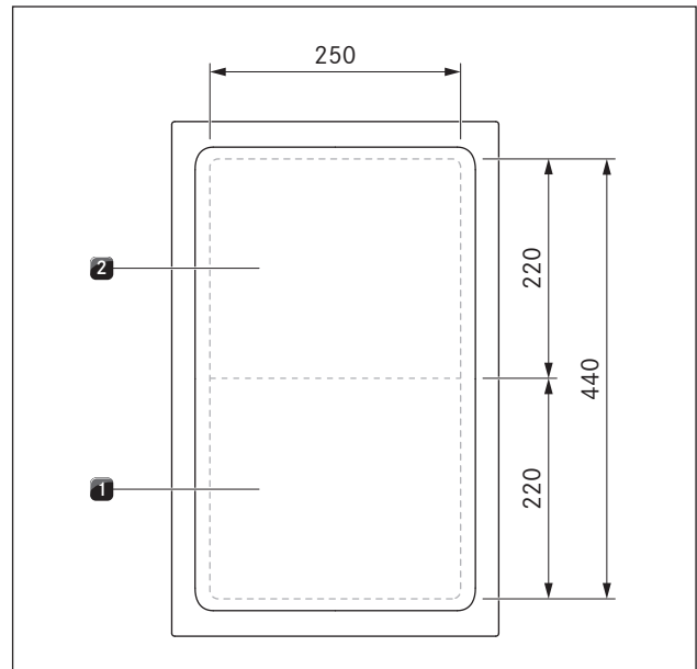
Afb. 4.17 Afmetingen kookzones
