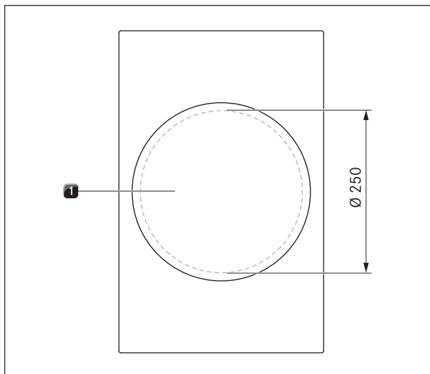
Afb. 4.11 Afmetingen kookzone
