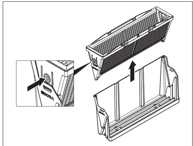
Afb. 6.3 Vetfilter verwijderen
