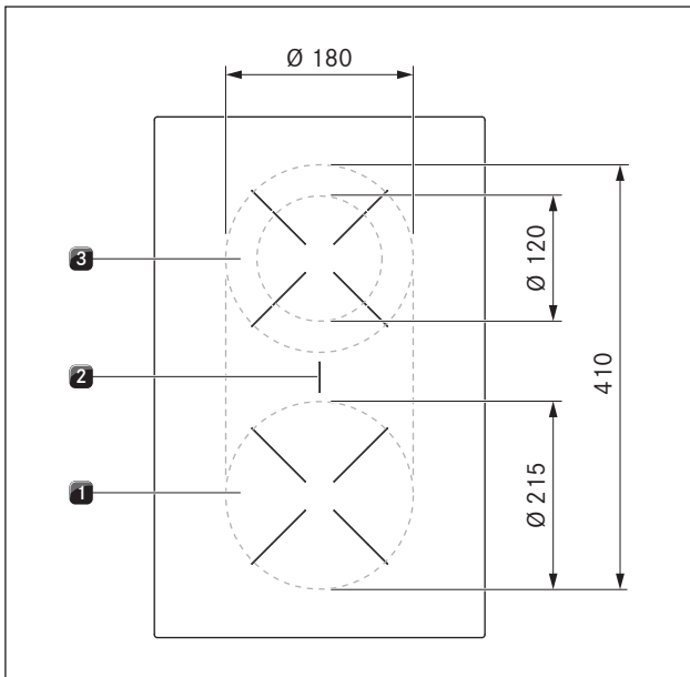
Afb. 4.15 Afmetingen kookzones
